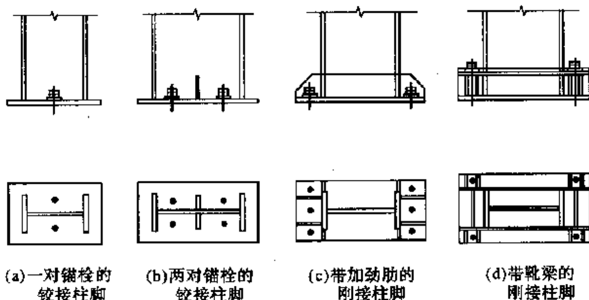
图 7.2.17 门式刚架轻型房屋钢结构的柱脚
