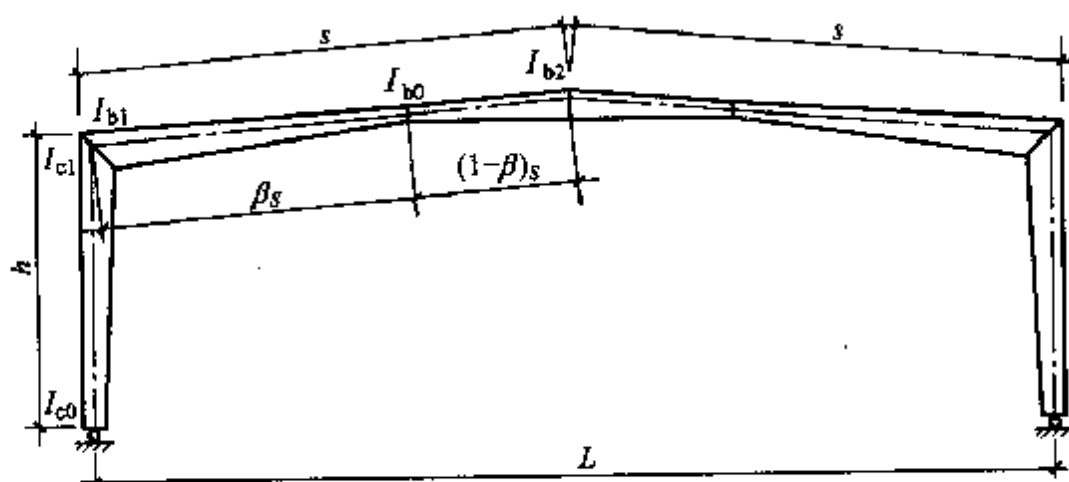
图 5.2.1 变截面刚架的几何尺寸
