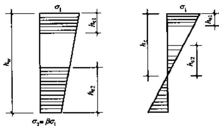
图 6.1.1 有效宽度的分布
