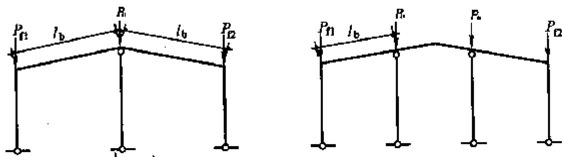
图 6.1.3-1 计算边柱时的斜梁长度
