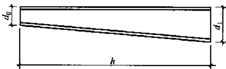
图 6.1.3-3 变截面构件的楔率
