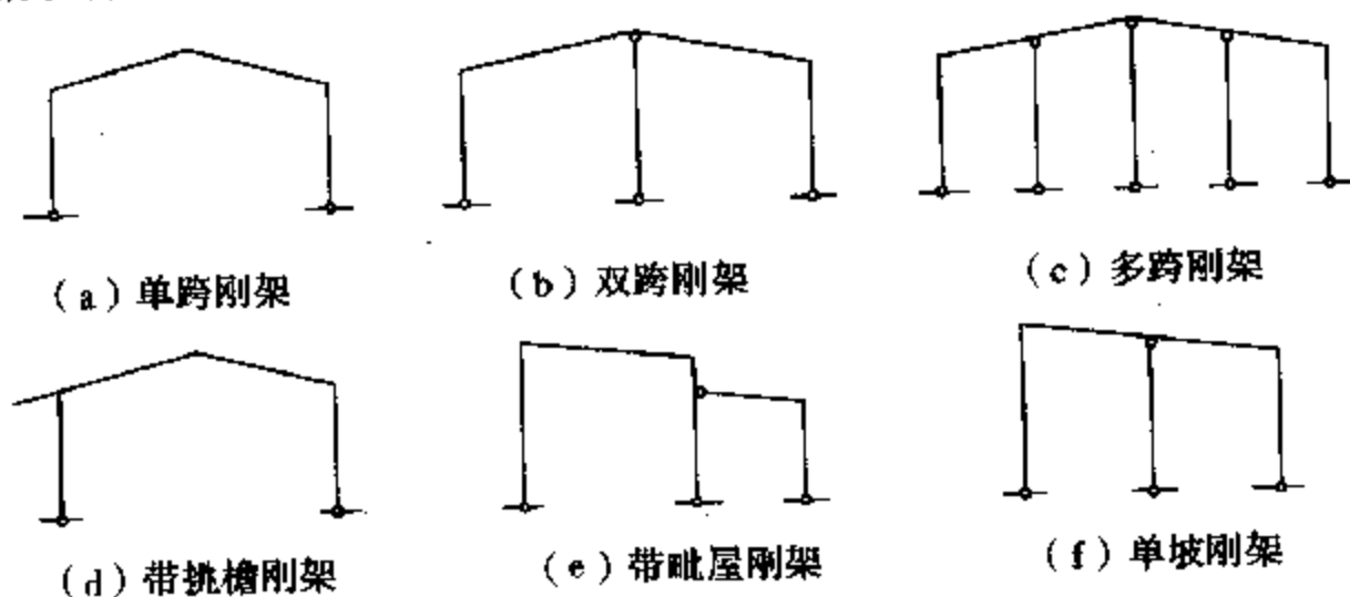
图 4.1.2 门式刚架形式示例
