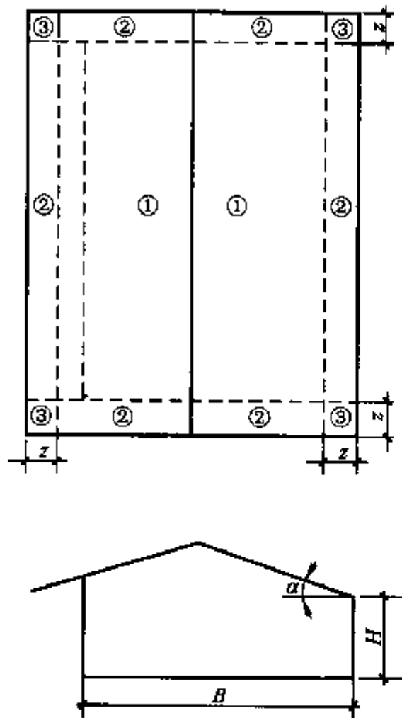
图 A. 0. 2-3 挑檐的风荷载体型系数分区
