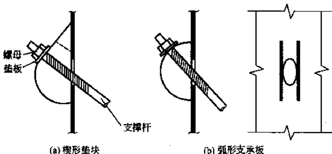
图 7.2.15 圆钢支撑的连接
