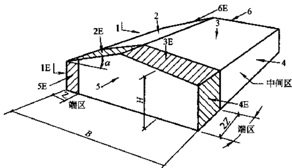
(a) 双坡刚架
