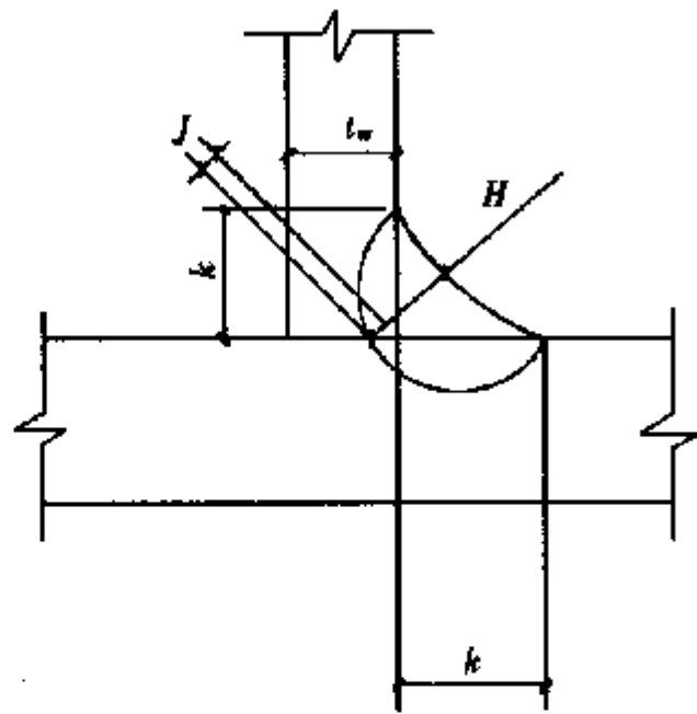
图 F.0.1 单面角焊缝
