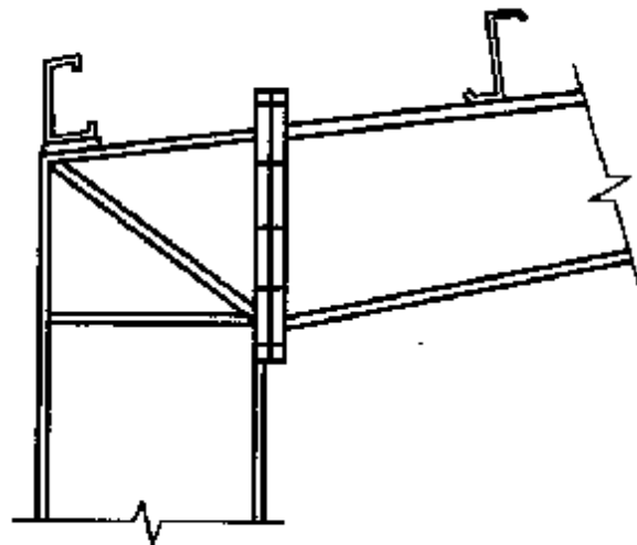
图 7.2.6 端板竖放时的螺栓和檩条
