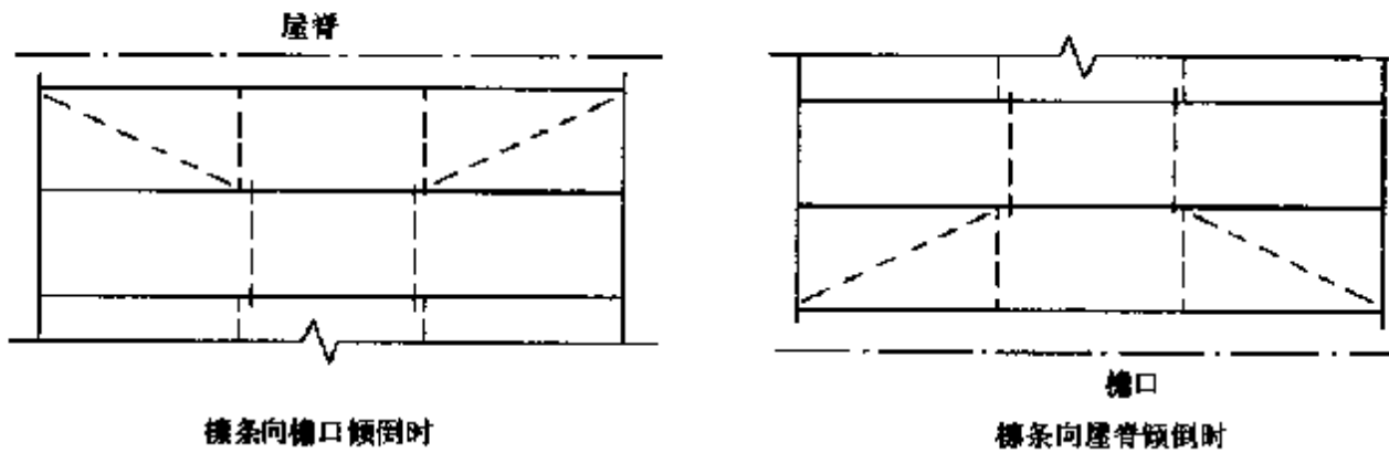
图 6.3.5 檩条间拉条的设置
