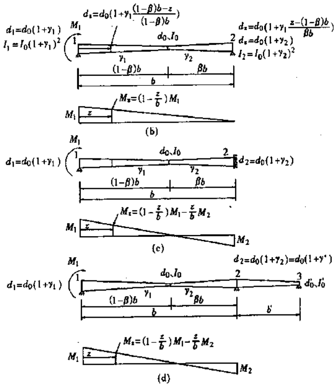
图 D. 0. 1-1 符号含义
