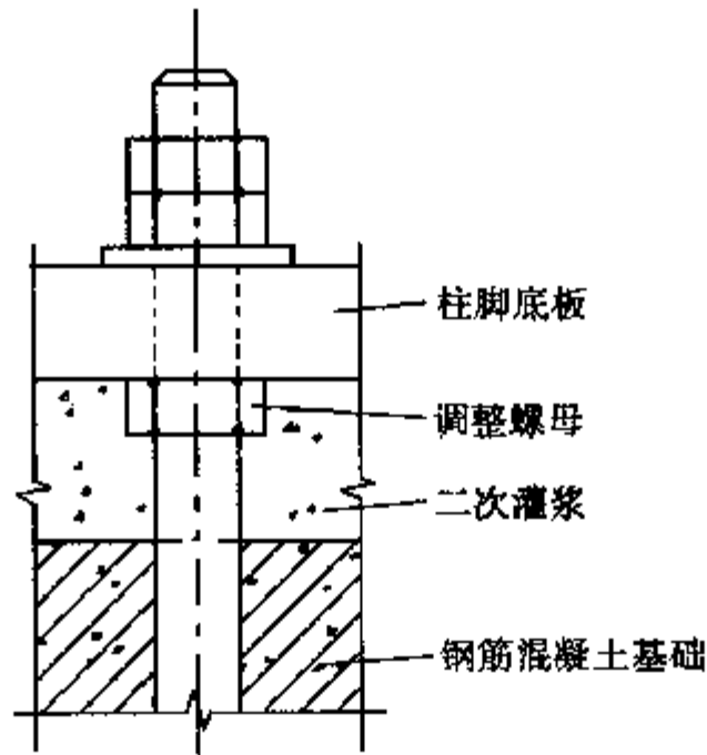
图 8.2.5 柱脚的安装
