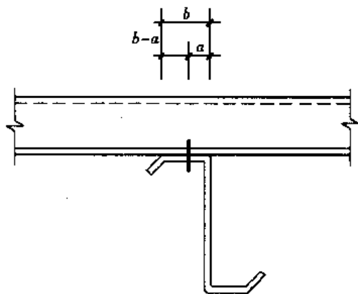
图 E.0.4 紧固件至转动中心的距离
