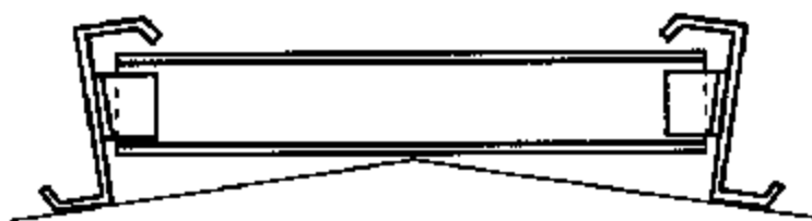
图 7.2.12 脊檩间的连系槽钢
