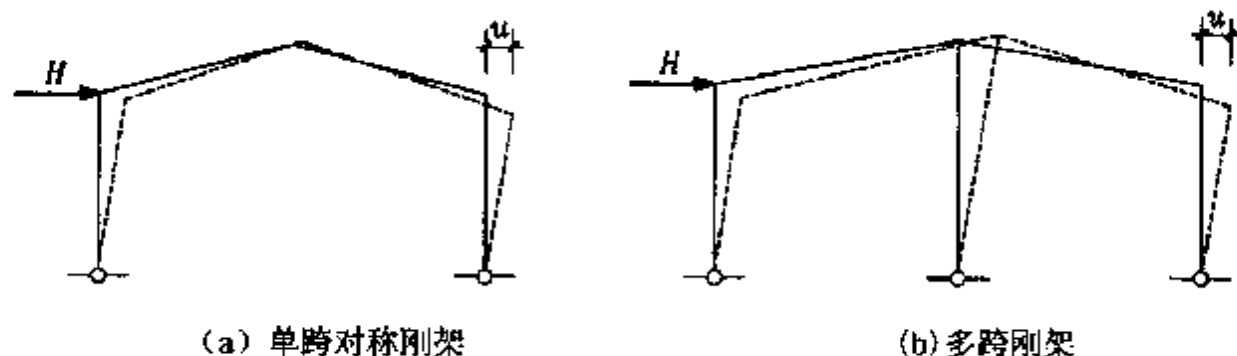
图 6.1.3-2 一阶分析时的柱顶侧移
