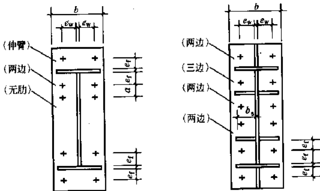
图 7.2.9 端板的支承条件
