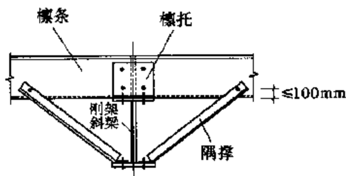
图 7.2.14 隅撑的连接
