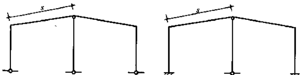
图 5.2.4 有摇摆柱的两跨刚架
