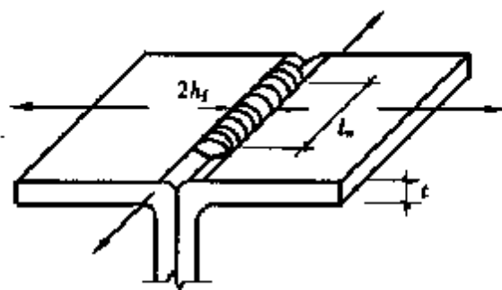
图 7.1.2-2 喇叭形焊缝
