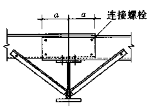
图 7.2.13 斜卷边檩条的搭接
