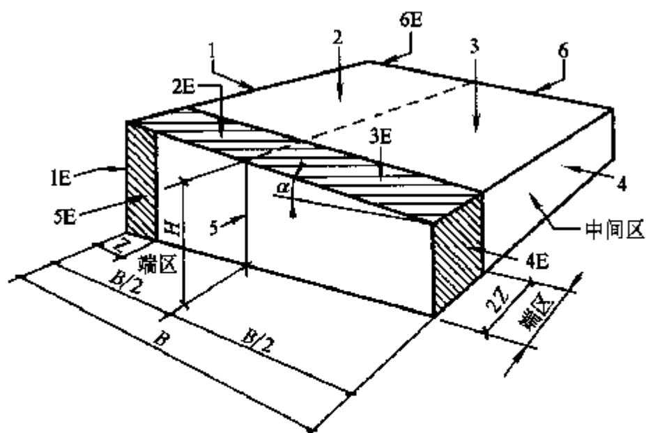
(b)单坡刚架
