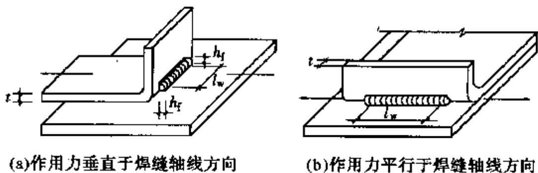
图 7.1.2-1 单边喇叭形焊缝
